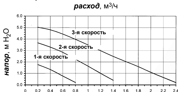
Рис. 12. Кривые расход/напор
