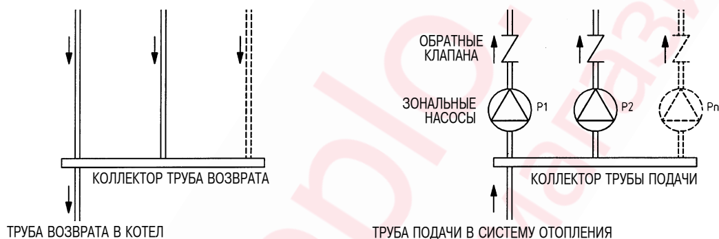
Рис.4. Гидравлические схемы для разветвленных систем
