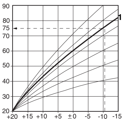
Рис. 8 Определение отопительной кривой
