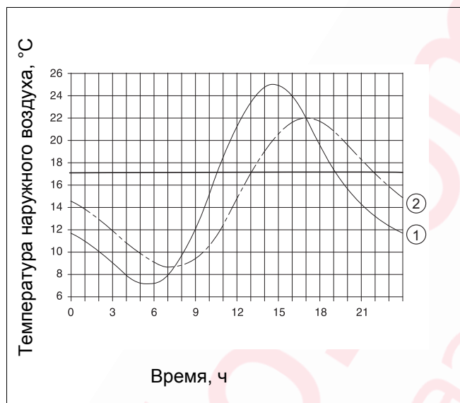
Рис. 7 Термическое запаздывание
