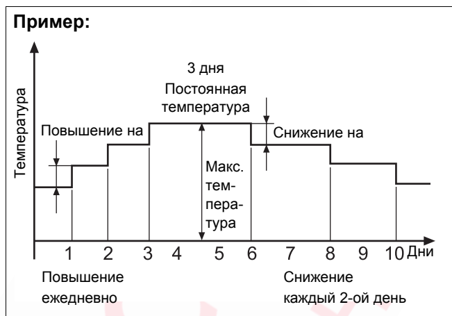
Рис. 13 Сушка пола
