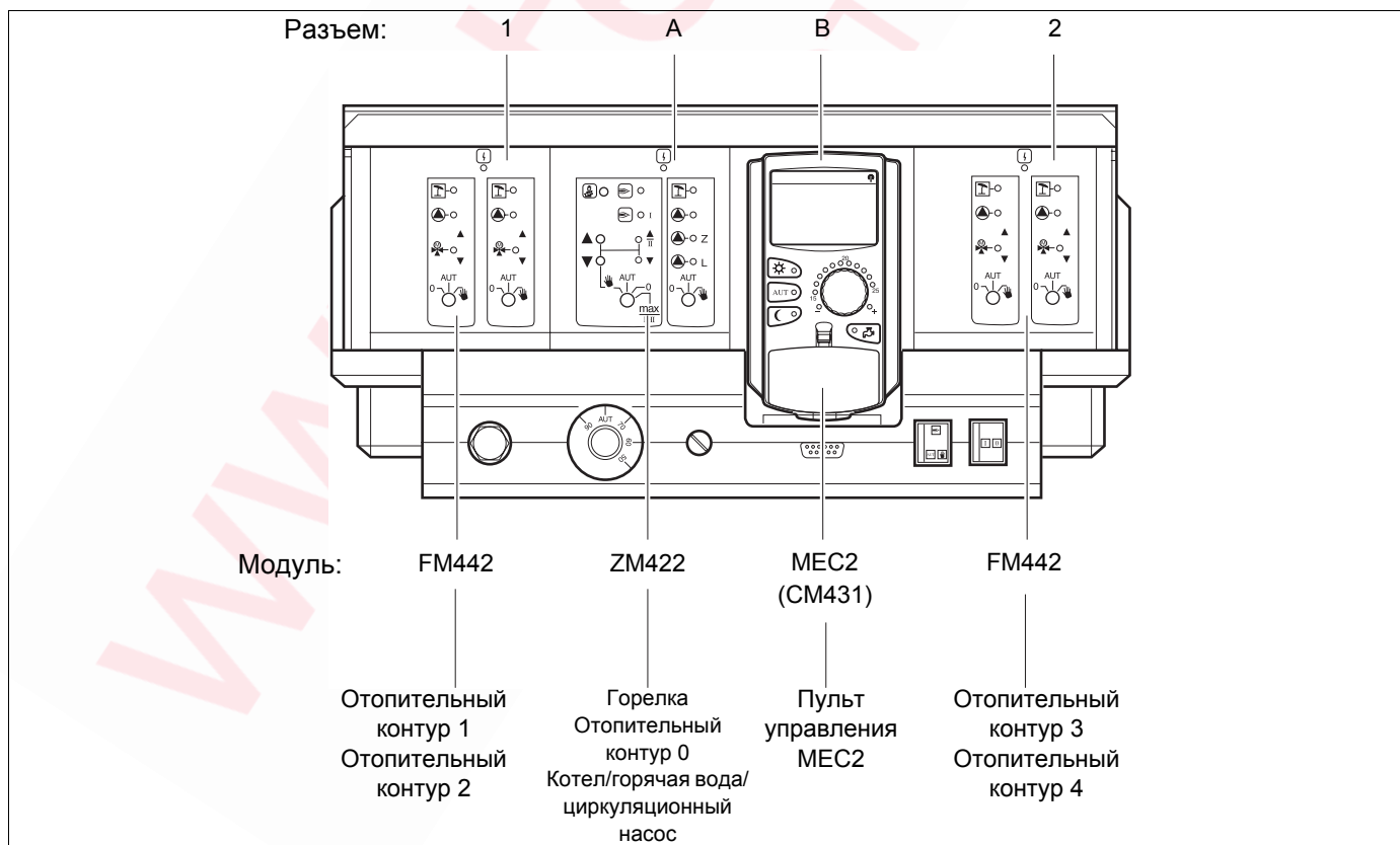
Рис. 7 Комплектация модулями
