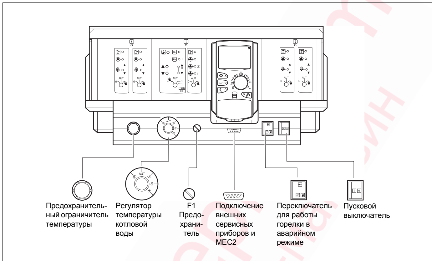
Рис. 6 Элементы управления
