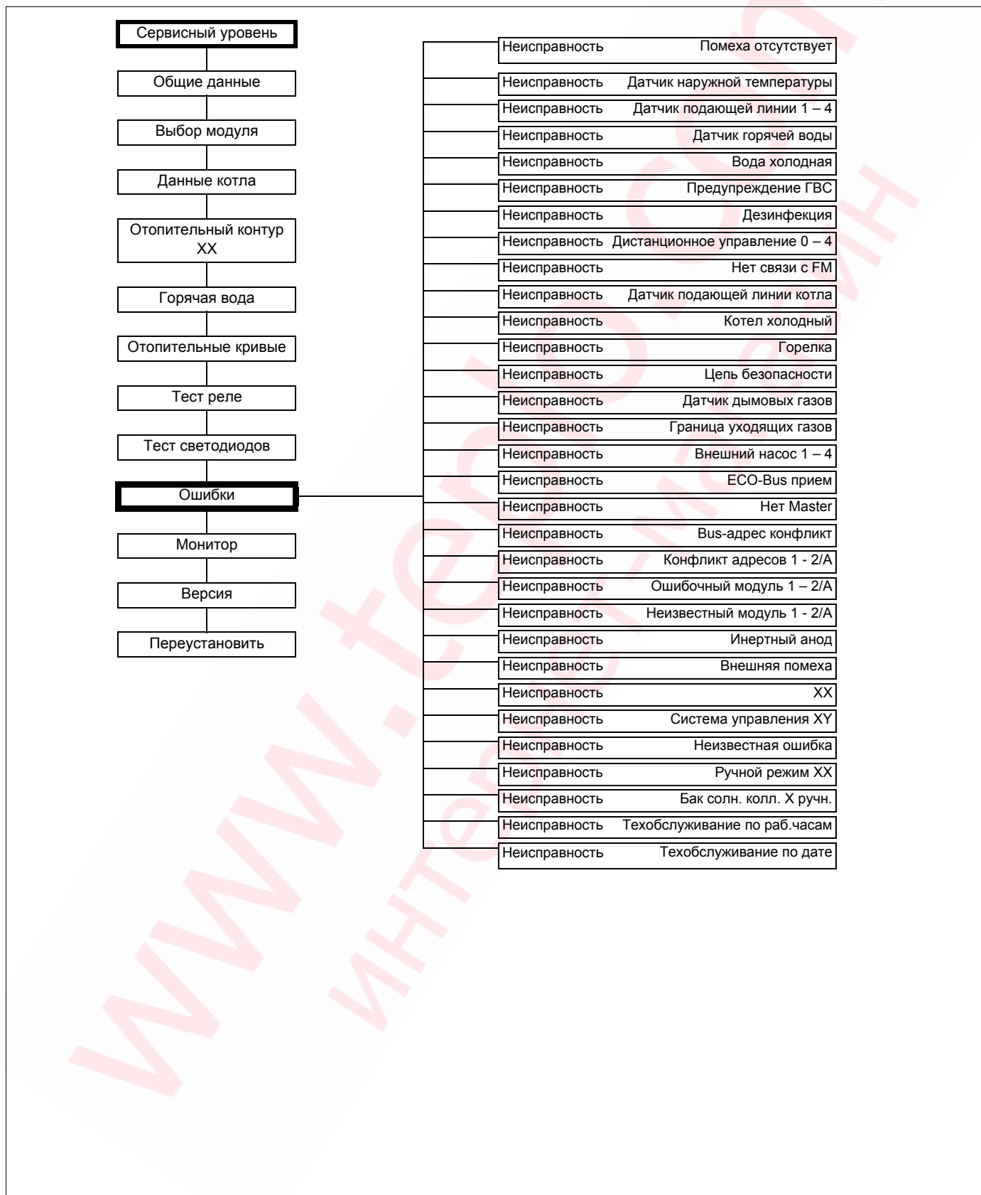
Рис. 16 Индикация неисправностей
