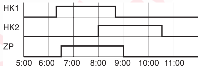
Пример программы циркуляционных насосов
