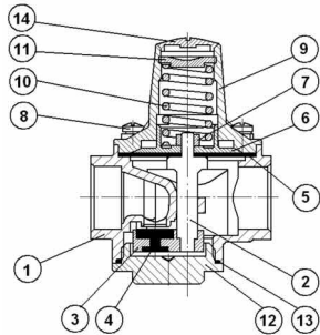
Рис. 1 Устройство редукционного клапана типа 7BIS.
