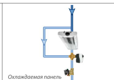
Охлаждаемая панель
