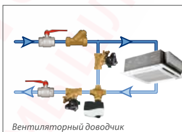
Вентиляторный доводчик
