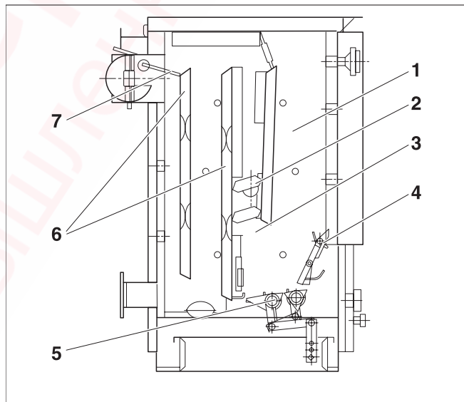
Рис. 2 Котел в разрезе, здесь тип K 24-1 S 61
