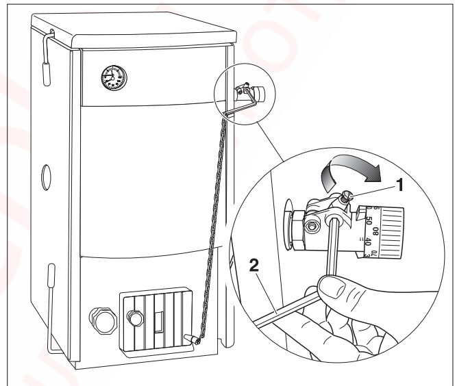
Рис. 7 Монтаж регулятора горения
