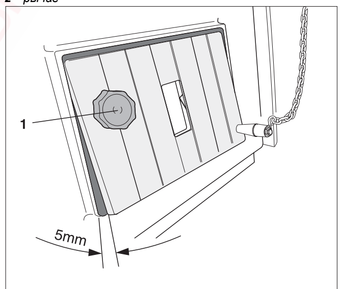
Рис. 8 Крепление цепи к воздушной заслонке
