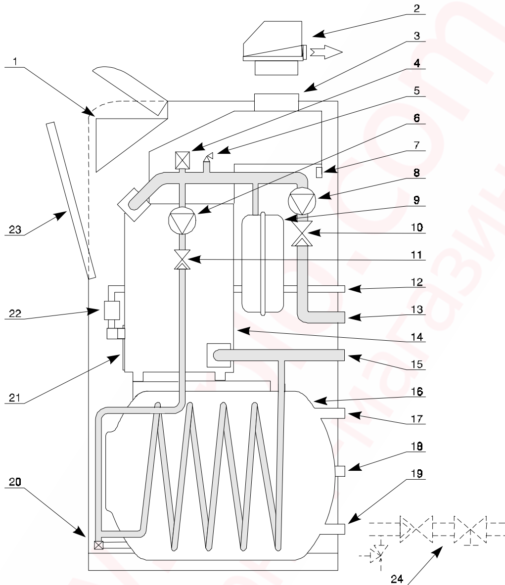
Рис. 2 Рабочая схема котла
