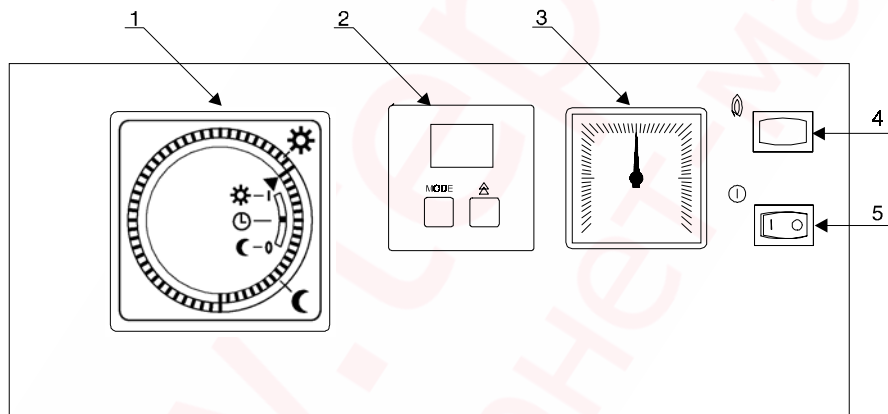
Рис. 3 Панель управления
