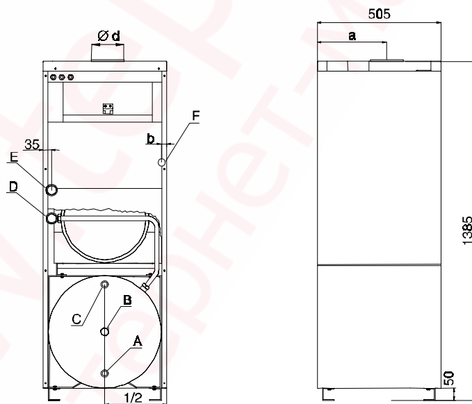
Рис. 1 Основные и присоединительные размеры
