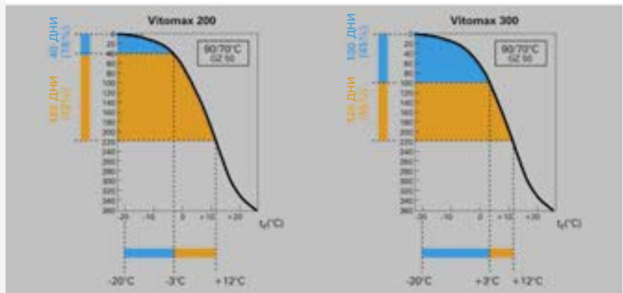
Сравнение диапазона погодной регулировки Vitomax 200 и Vitomax 300
